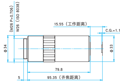
PFL-20-UV-AG-LC11-A
